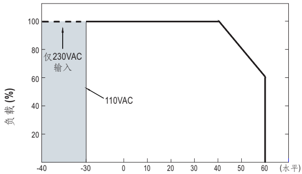
环境温度, Ta (°C)
