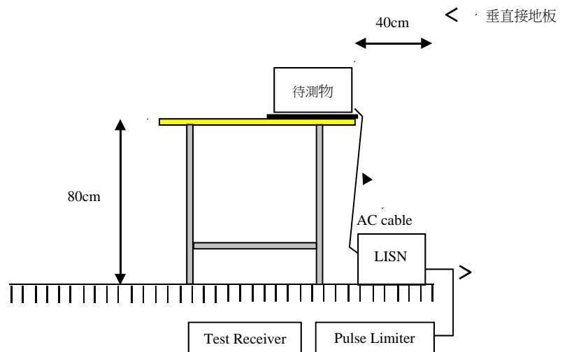
圖一: 明緯EMI 測試系統配置圖
