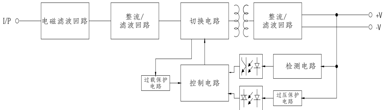
■ 方框图
