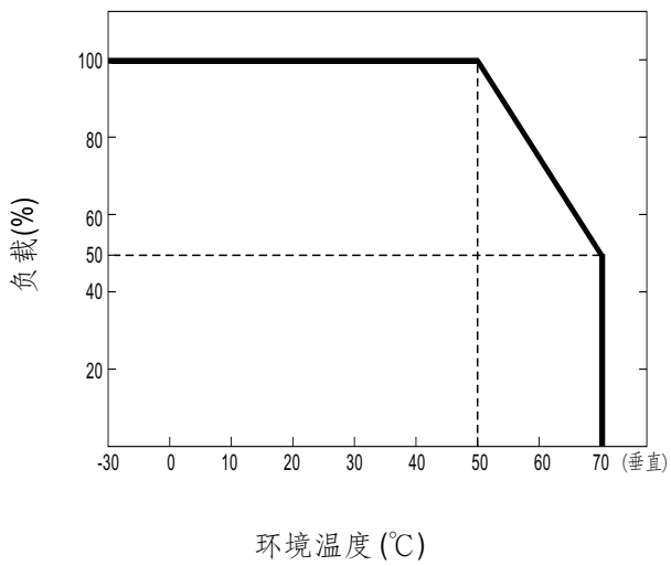
■ 减额曲线
