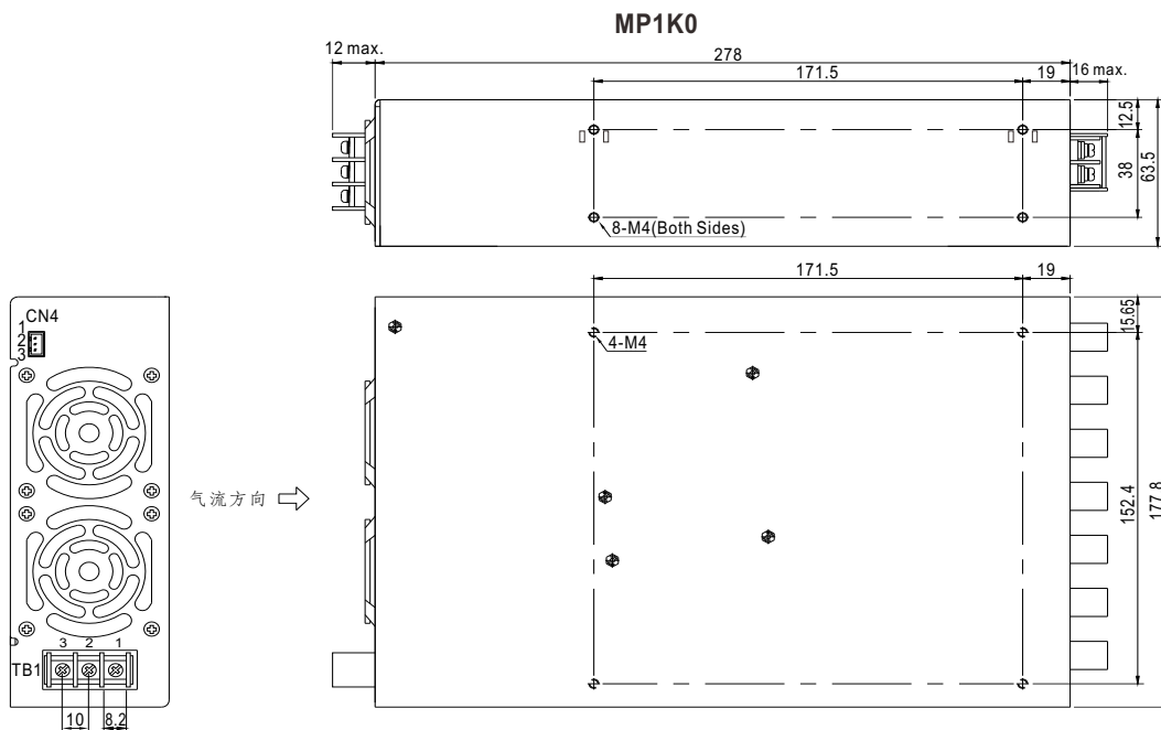
TB1(PFC-450/650/1K0)
