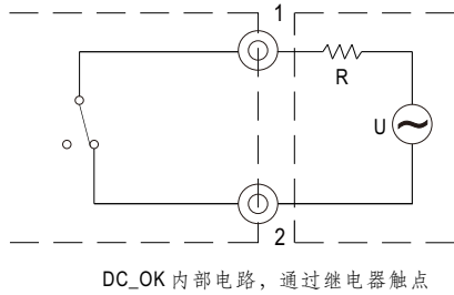
外部电压源(U)和电阻(R) (最大电流源为 30Vdc/1A、30Vac/0.5A)
