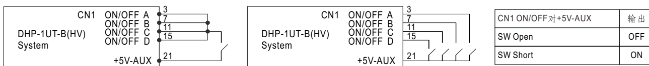
图 4-1 遥控器连接
