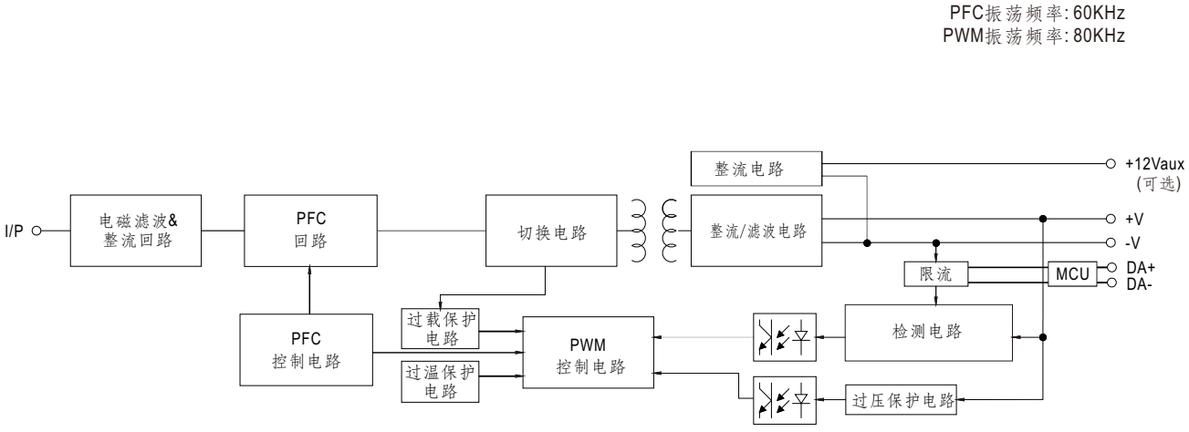
■ 方框图
