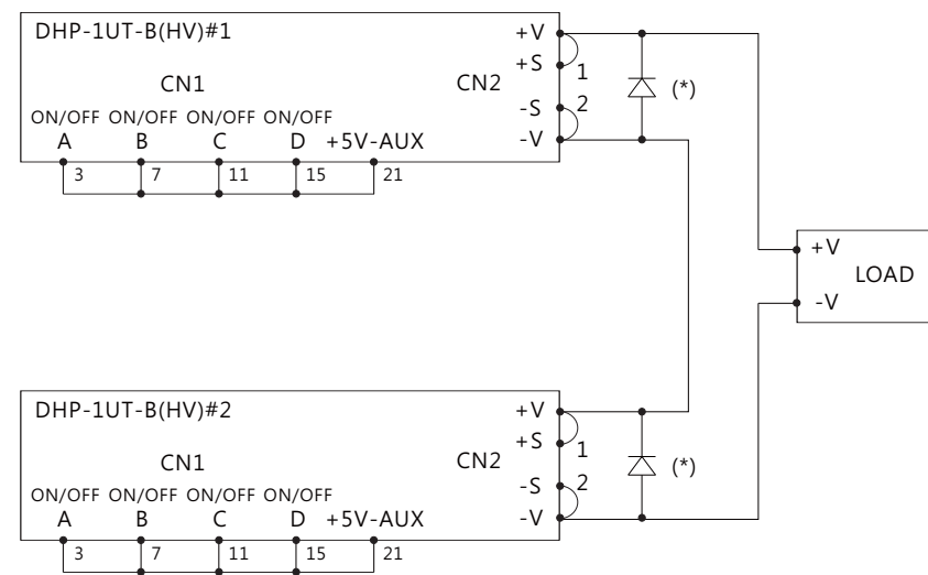
圖5-11 串聯操作配置方式示意圖
