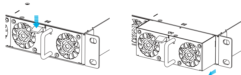
圖3-3 NCP-3200取出機箱示意圖
