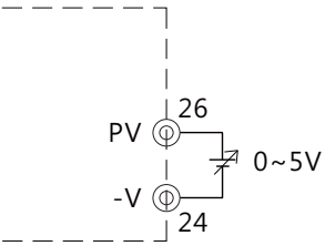
圖5-1 外加直流電壓連接方式
