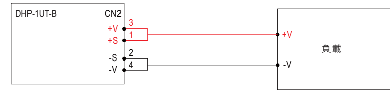
圖5-9 Local Sense配線示意圖
