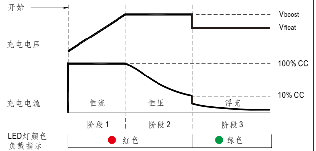
◎ 3 段式充电曲线
