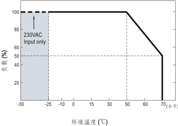
■ 减额曲线
