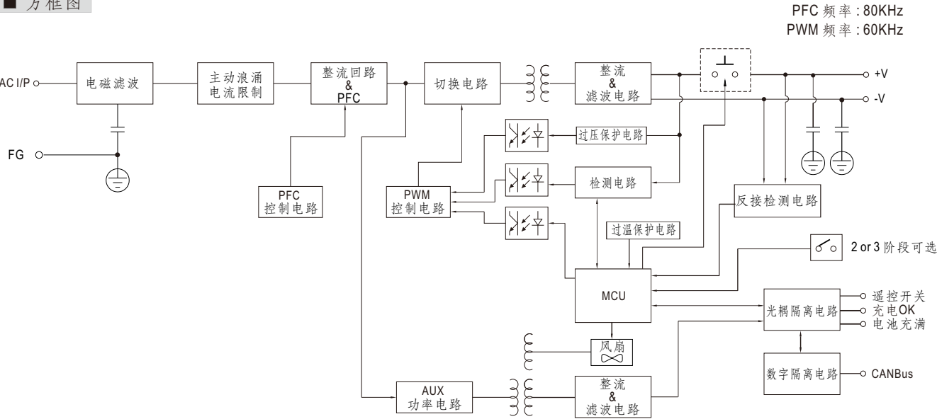
■ 方框图
