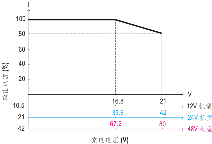
■ 减额曲线
