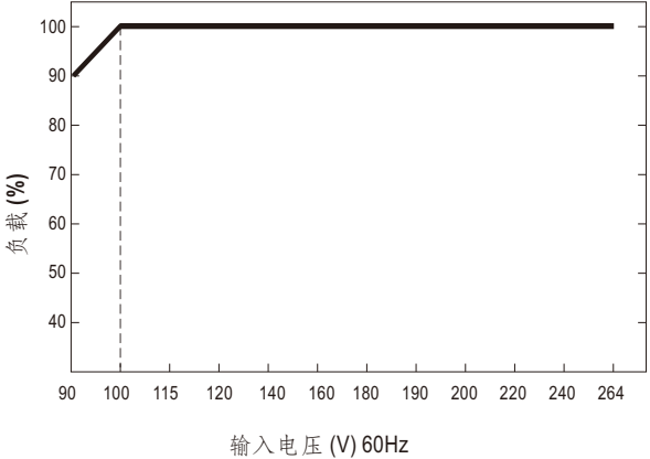
■ 静态特征曲线
