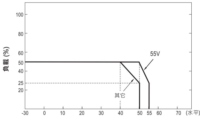
使用2個 85CFM 風扇的環境溫度
