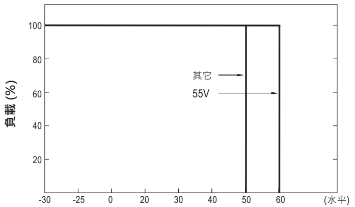
Tcase (°C)
