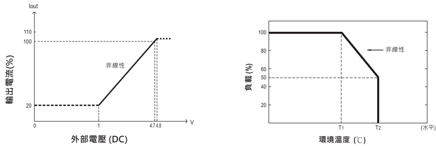
◎ 150A/87A/46.3A/30A輸出電流為100%
