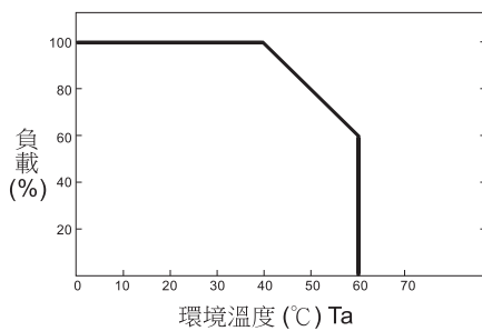
圖7.2 輸出減額曲線圖
