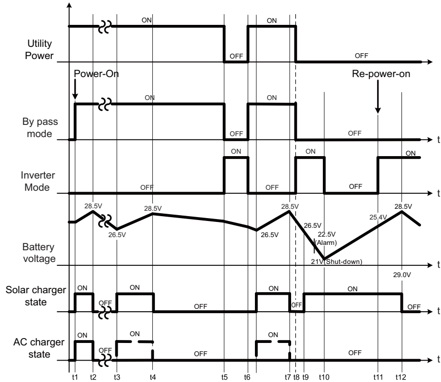
圖4.1 UPS模式程序控制圖
