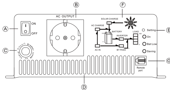
圖3.1 前面板示意圖(TN-1500)
