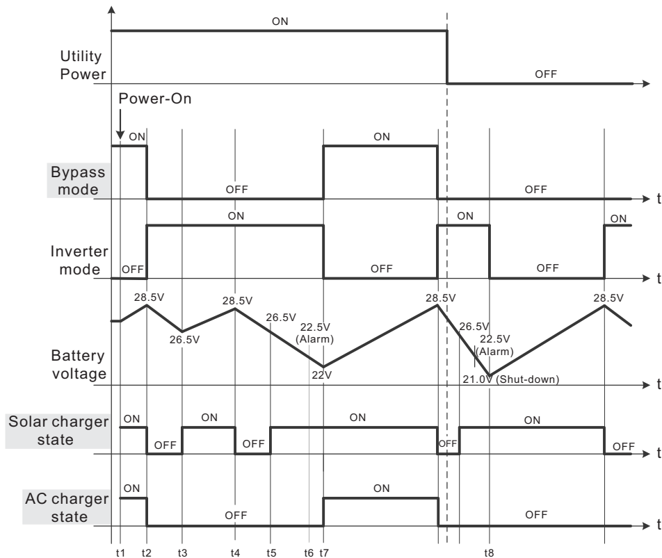
圖4.2 節能模式程序控制圖
