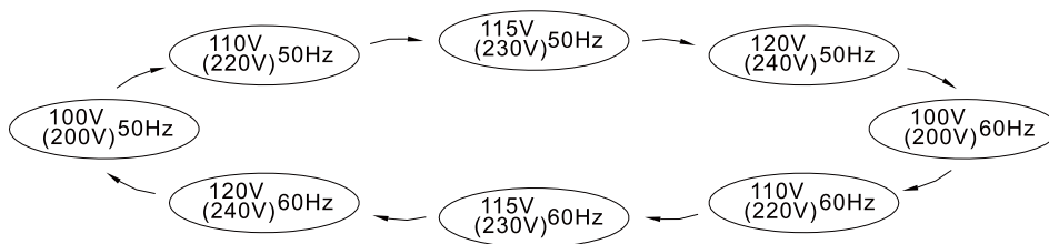
圖5.2輸出電壓、頻率設定變換順序圖
