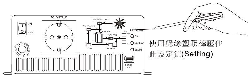
圖5.1 輸出電壓、頻率及省電模式調整示意圖
