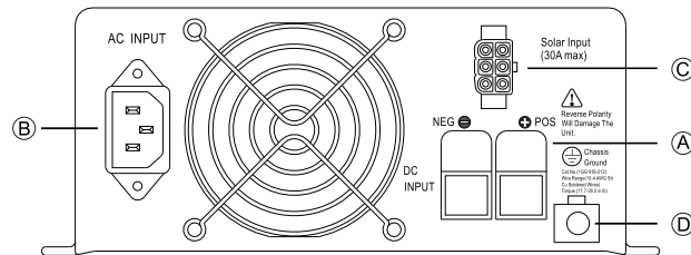
圖3.2 後面板示意圖(TN-1500)
