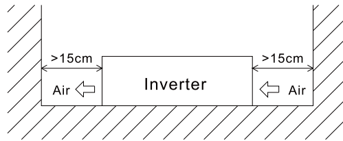
圖7.1 固定示意圖
