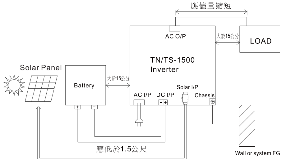
圖7.1 固定示意圖
