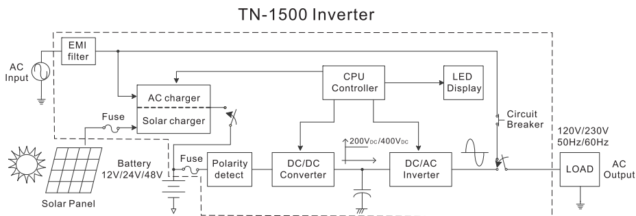
圖2.1 系統方塊圖
